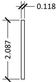
3 FIN
